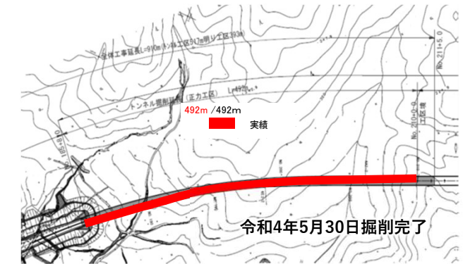
トンネル進捗図
