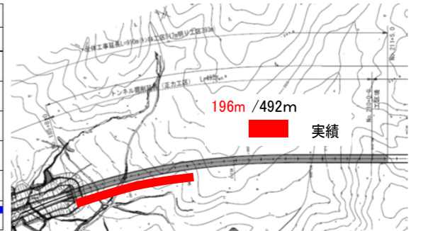
トンネル進捗図 12/25現在
