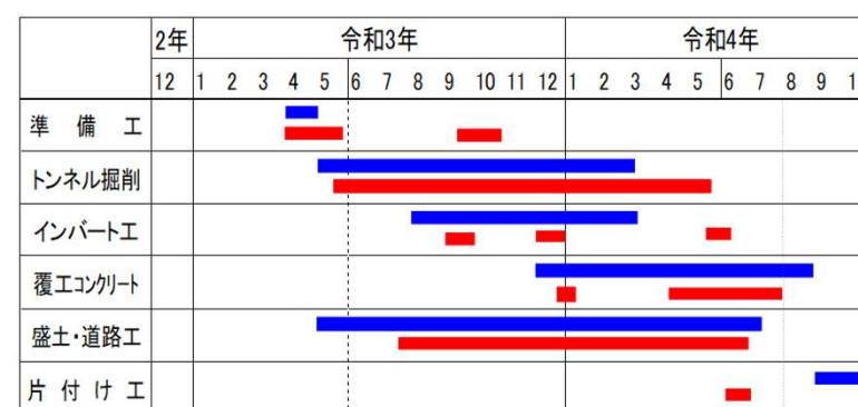
全体工程表
