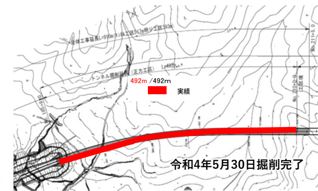
トンネル進捗図
