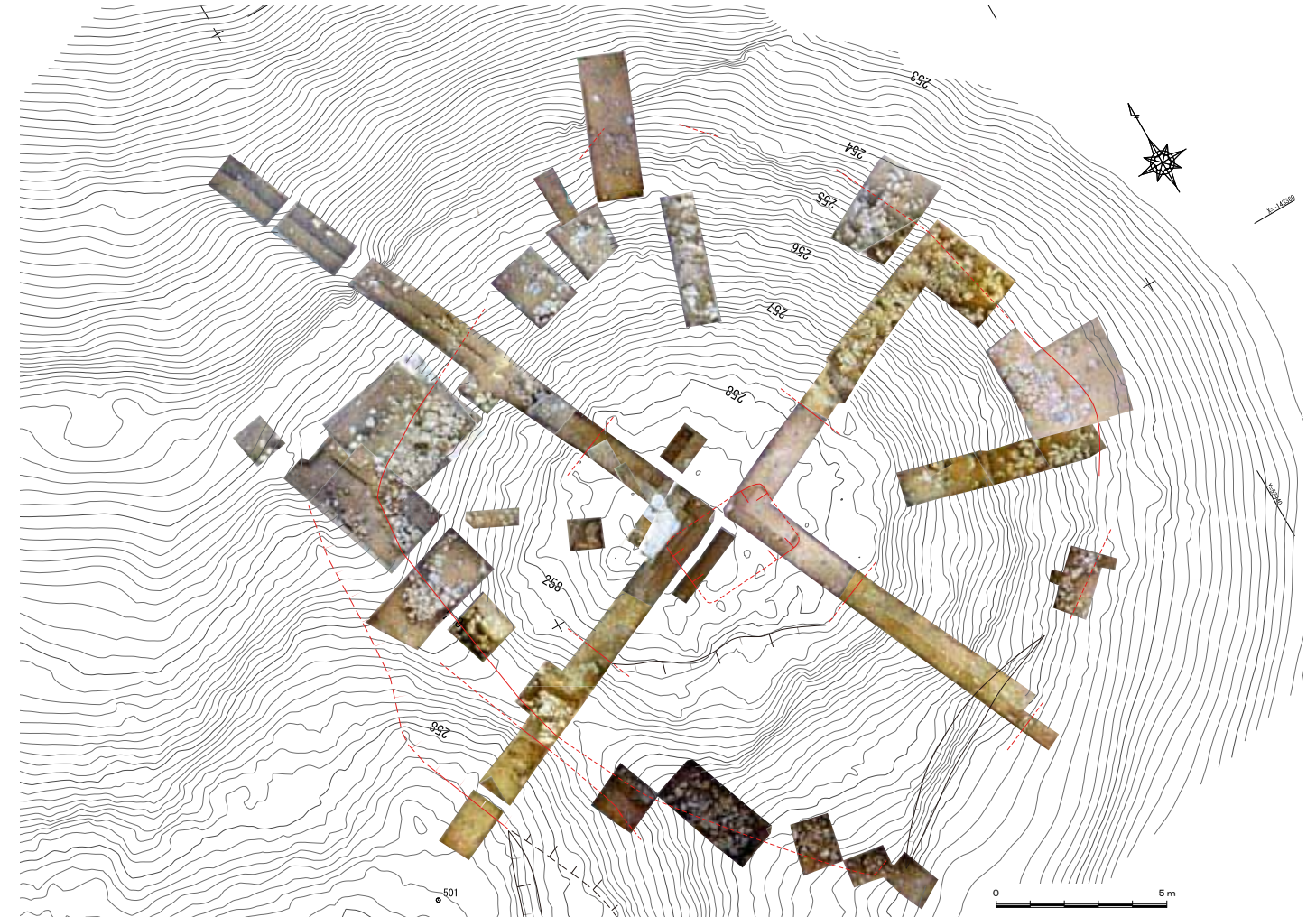
甲立第2号古墳墳丘測量図（S = 1 : 200）
