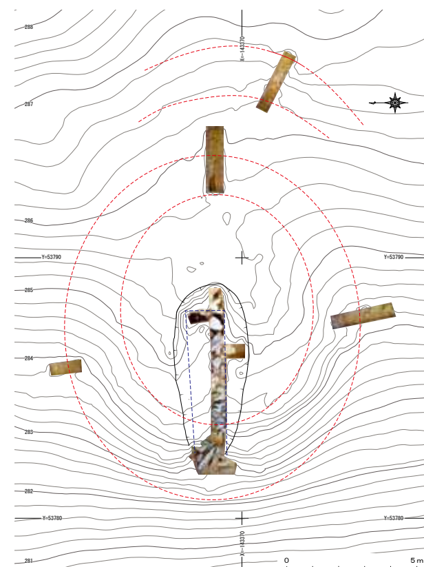
甲立第3号古墳墳丘測量図（S = 1 : 200）
